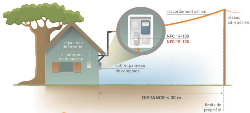
T1 RACCORDEMENT TYPE 1 AÉRIEN < 30 m
