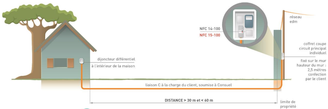
T2 RACCORDEMENT TYPE 2 AÉRIEN > 30 m ET < 60 m
