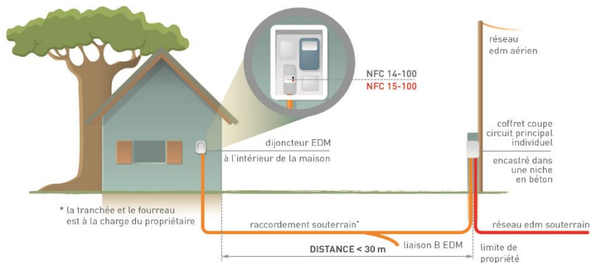
T1 RACCORDEMENT TYPE 1 AÉRO-SOUTERRAIN OU SOUTERRAIN < 30 m
