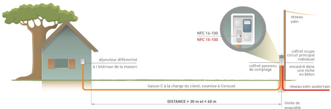
T2 RACCORDEMENT TYPE 2 AÉRO-SOUTERRAIN OU SOUTERRAIN > 30 m ET < 60 m
